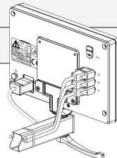
Soporte multiposición (1197273-02)
